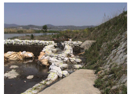
芥川大橋上流土嚢による実験魚みち作り(06.5.3)
